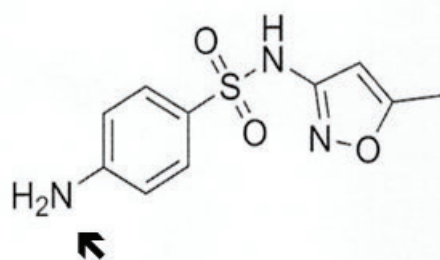
Sulfamethoxazole
